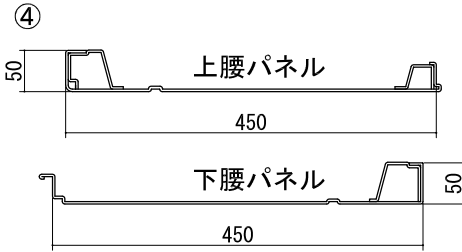
腰パネル t=0.6
