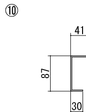
妻板 t=0.7
