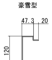
母屋 t=2.3
