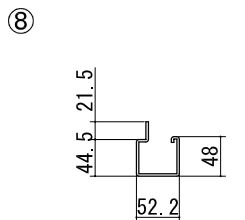
軒とい t=0.6
