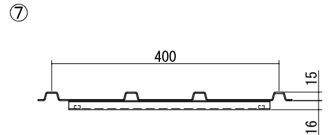
母屋 t=1.6
