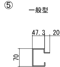
母屋 t=1.6
